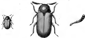
Cryptocephalus tridentatus.
